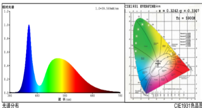
光谱分布
